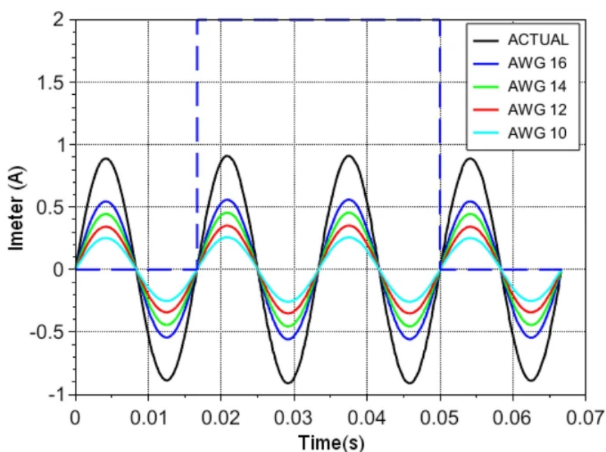
Simulované priebehy prúdu v inteligentnom merači pri rôznych hodnotách odporu bypassu
