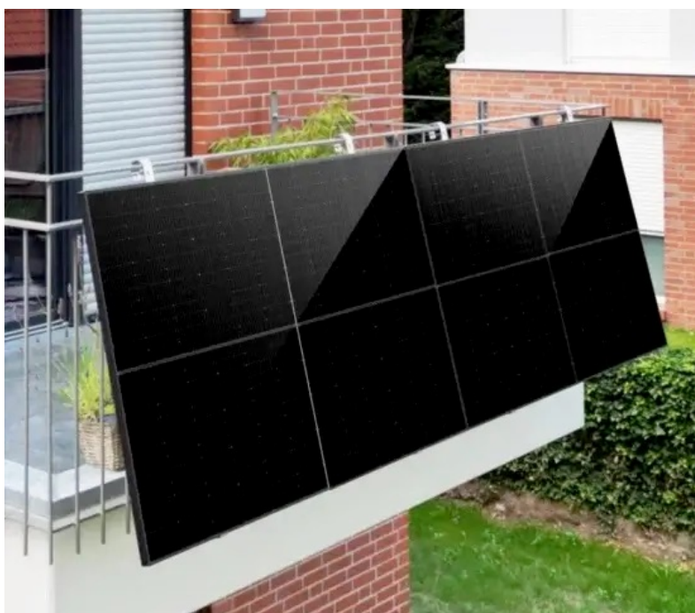
Balkónový integrovaný fotovoltaický systém obsahuje: 2 solárne panely o celkovom výkone 800 W, monitorovaciu jednotku, káble na pripojenie a mikroinvertor
