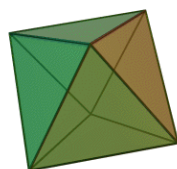
Oktaéder
