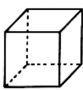
Kocka
