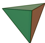
Tetraéder
