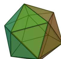
Ikosaéder
