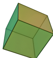
Hexaéder
