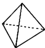
Štvorsten
