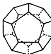
Dvanásťsten
