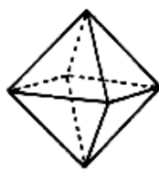
Osemsten
