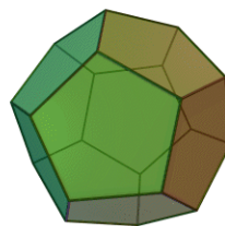
Dodekaéder
