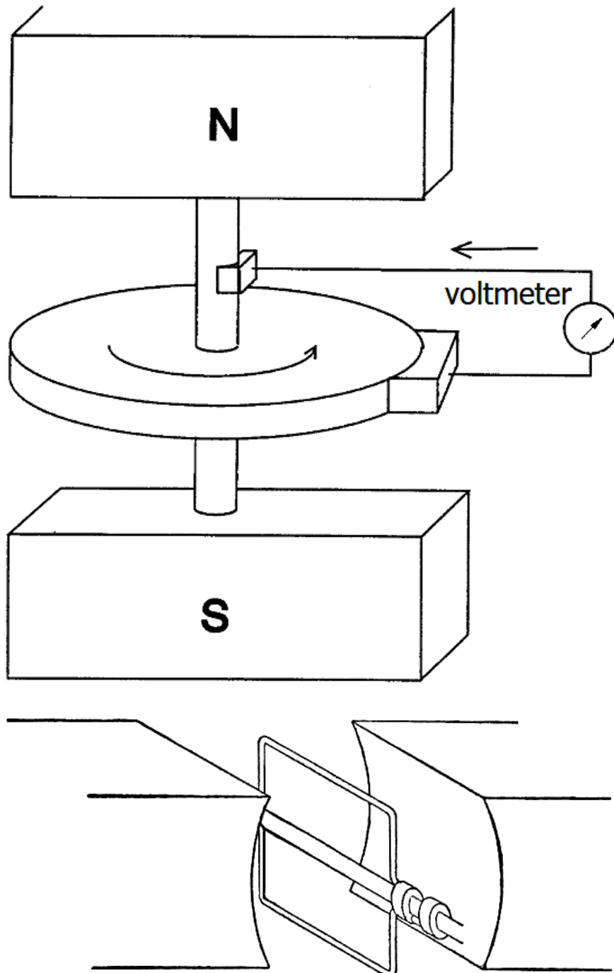
Princíp dynama
