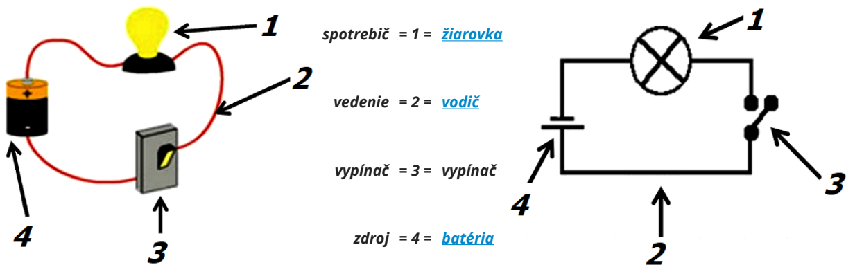
Prevodník pojmov jednoduchého elektrického obvodu
