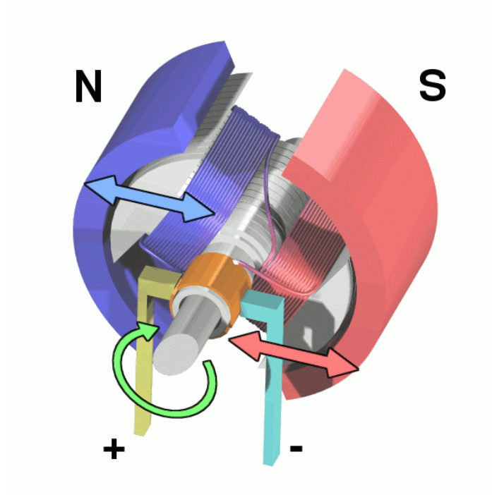
Princíp práce jednosmerného elektromotora
