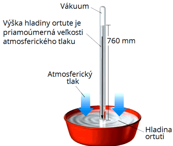
Princíp práce barometra
