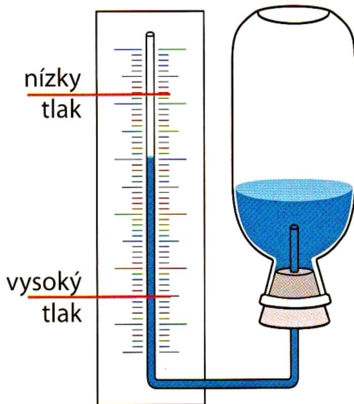
Doma vyrobený barometer
