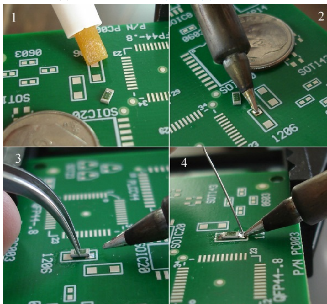
Montáž SMD súčiastok
