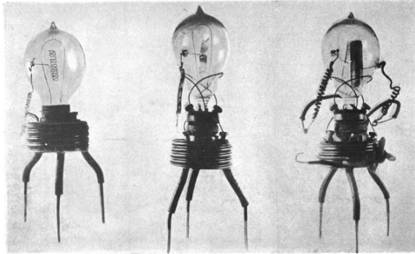
Prvý prototyp Flemingovej elektrónky z roku 1904
