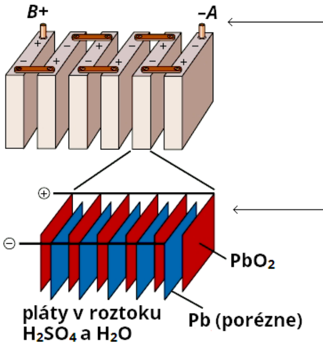
Olovený akumulátor
