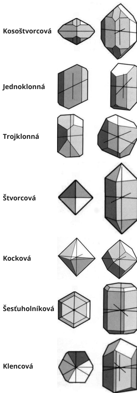
Kryštálové sústavy
