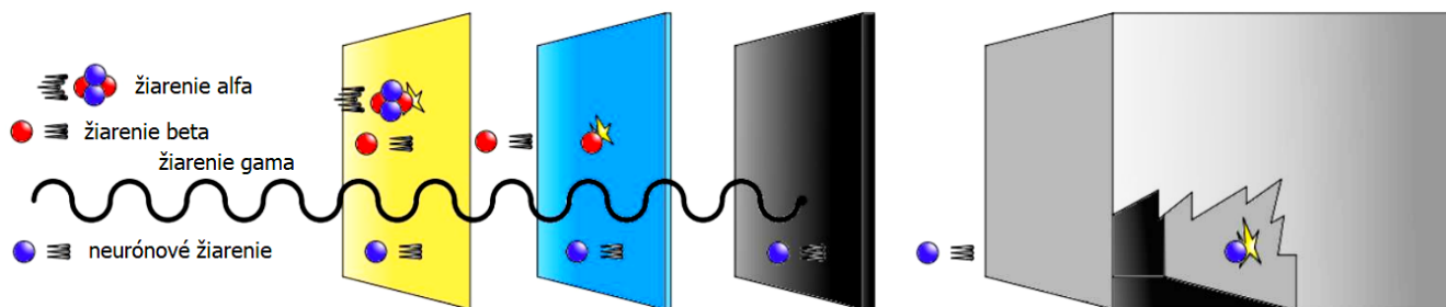
Druhy žiarenia a ich prenikavosť
