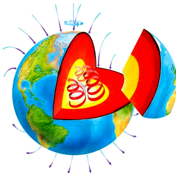
Magnetické pole Zeme
