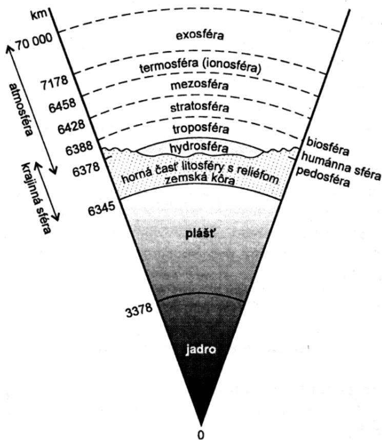
Vertikálny prierez Zemou
