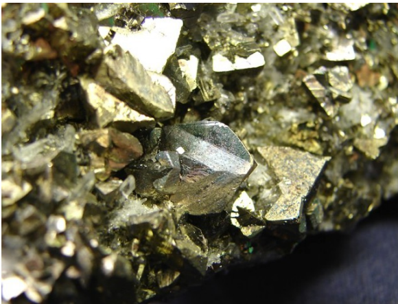
Sulfid meďnato-železnatý
