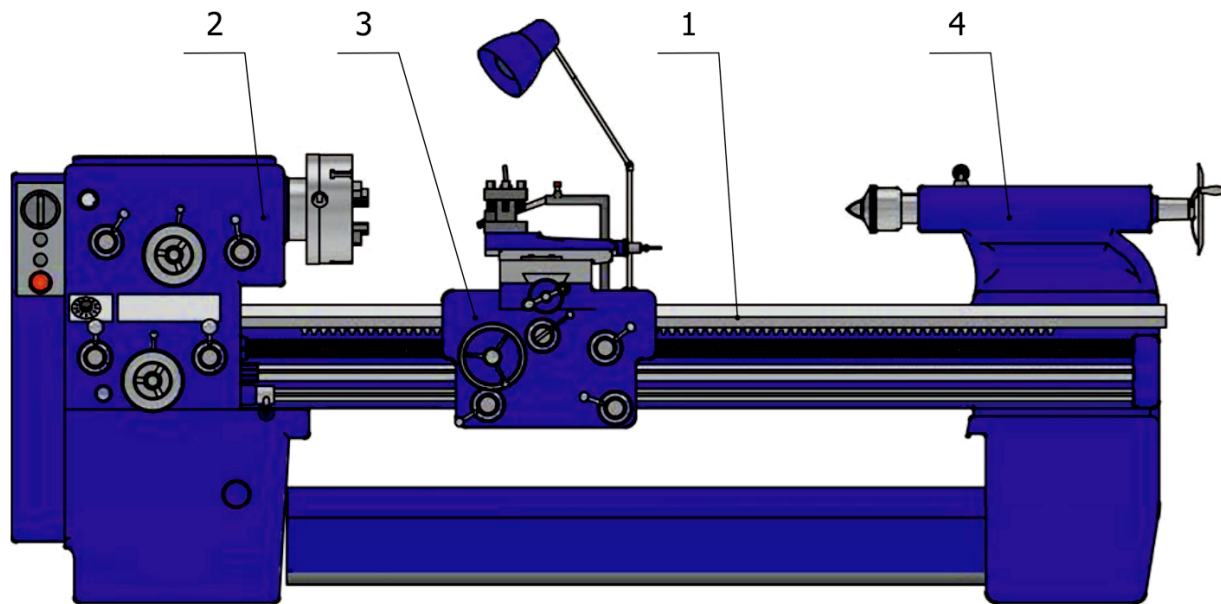
Hrotový sústruh: 1 - lôžko, 2 - vreteník, 3 - suport, 4 - koník
