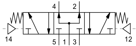
5/3 ventil so strednou polohou zavzdušnenou
