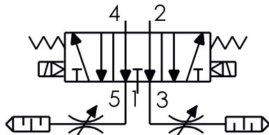
5/3 e-ventil, v strednej polohe prípojky odvzdušnené
