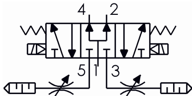
5/3 e-ventil, v strednej polohe prípojky pod tlakom
