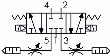
5/3 ventil, v strednej polohe prípojky uzavreté
