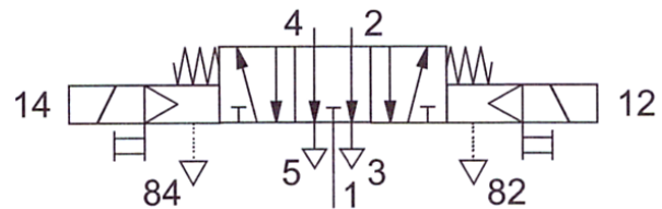
Nepriamo riadený 5/3-cestný ventil v kľudovej polohe otvorený
