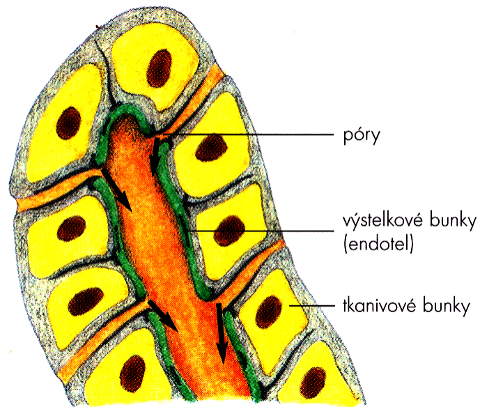
Schématický prierez miazgovou kapilárou
