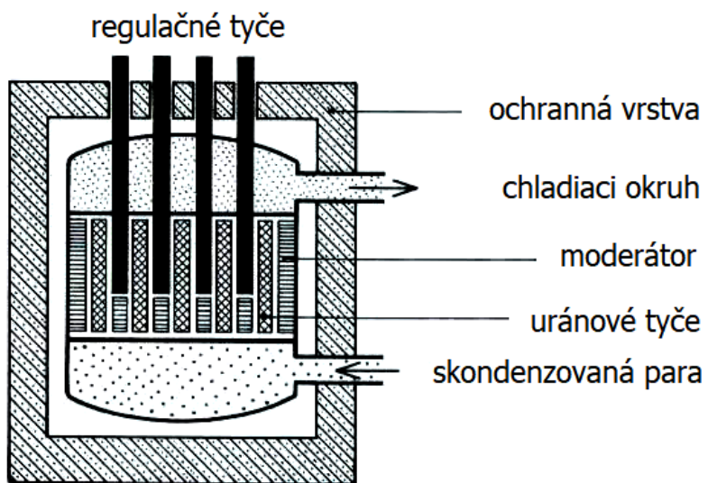
Jadrový reaktor
