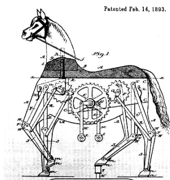
Patent na mechanického koňa
