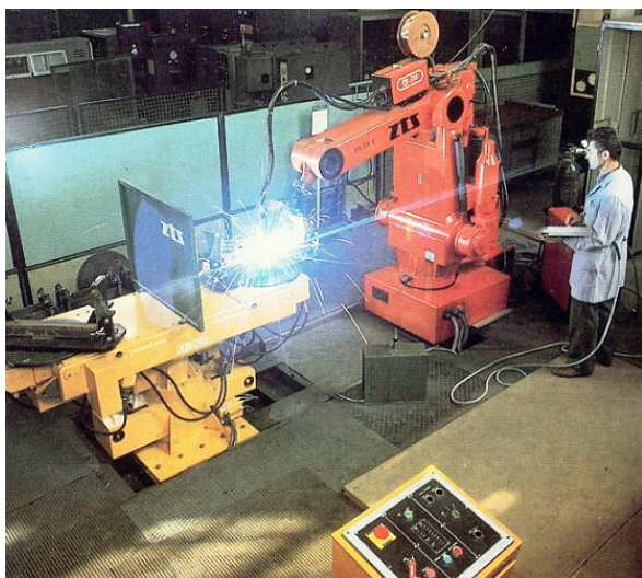
Pracovisko na oblúkové zváranie s robotom PR 32-E a polohovadlom DOM 200 vo Výskumnom ústave zväračskom v Bratislave
