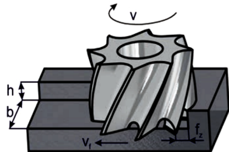
Čelné frézovanie
