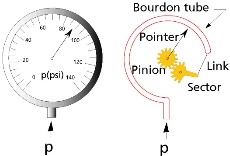
Konštrukčná schéma deformačného manometra s Bourdonovou trubicou v tvare písmena C (1 psi = 6894,8 Pa, 1 Pa = 0,000145 psi)
