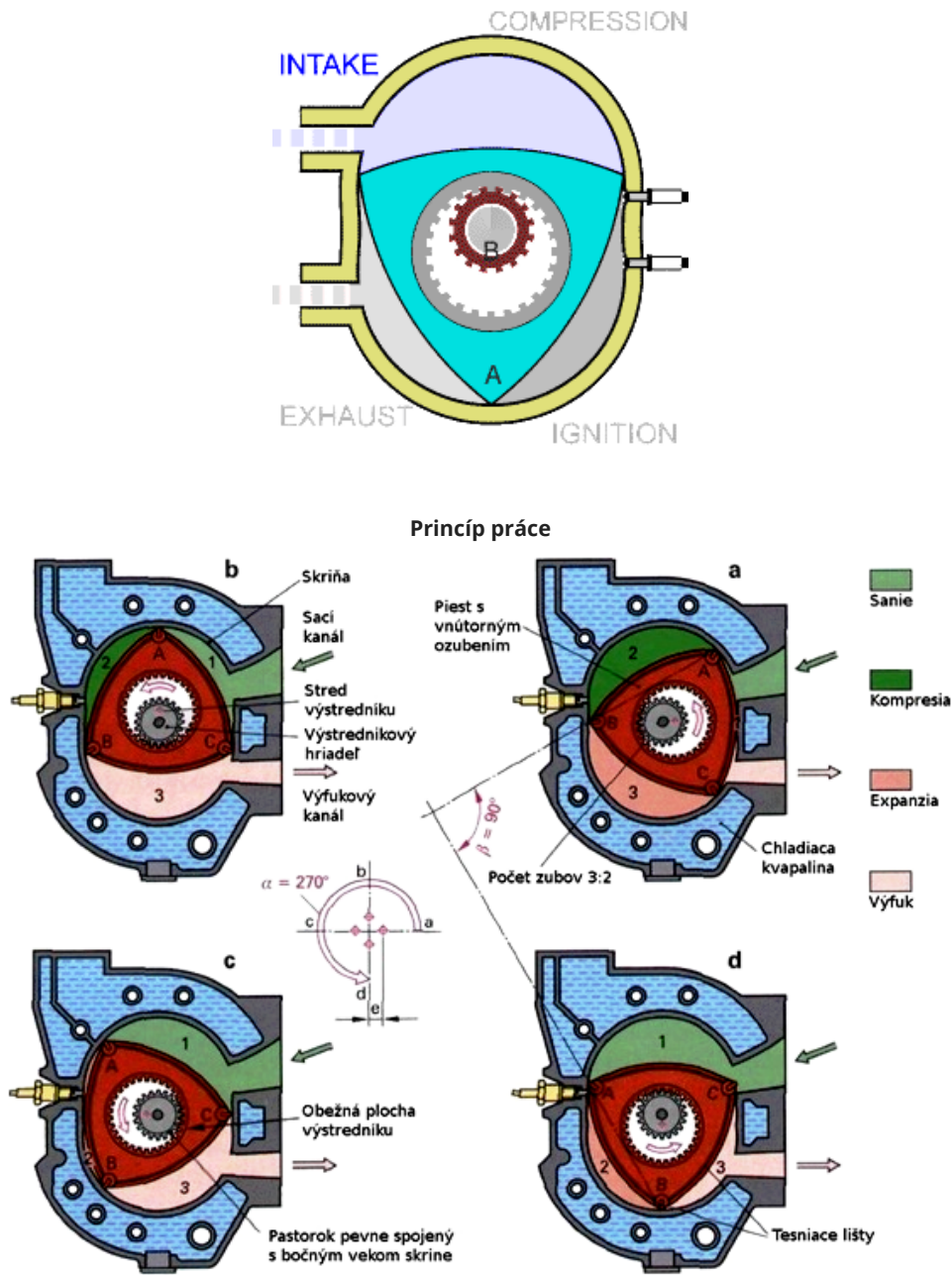
Zloženie a princíp práce Wankelovho motoru
