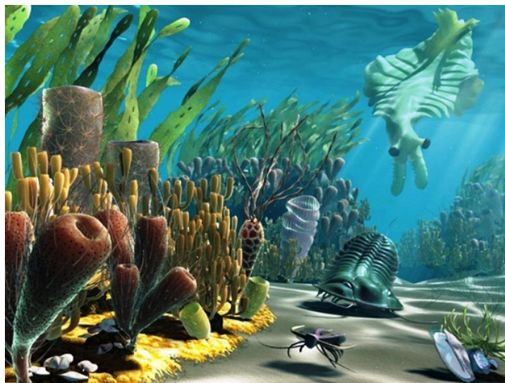
Kambrium
