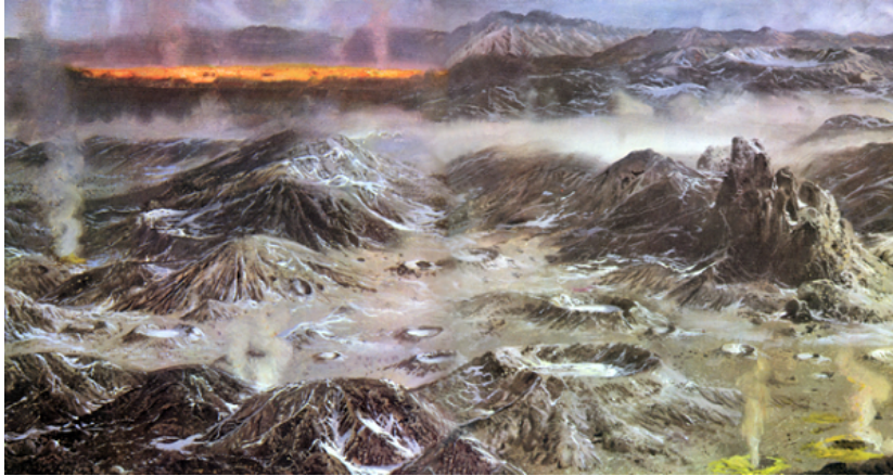
Prahory
