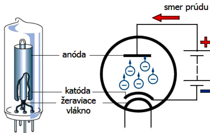
Elektronková dióda
