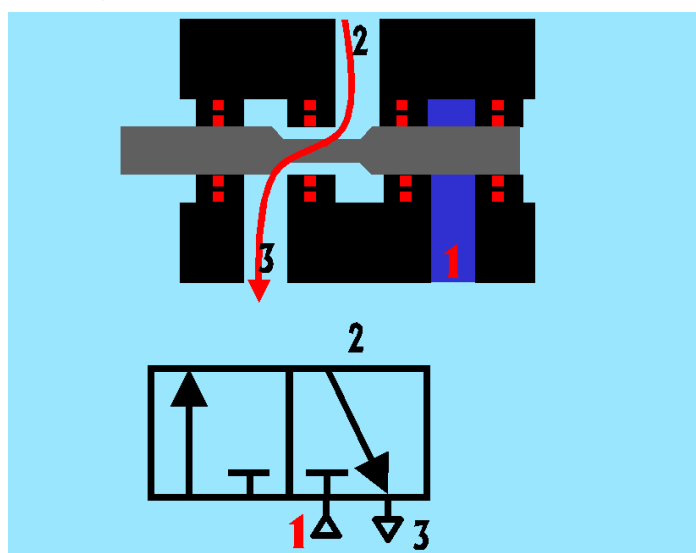
3/2-cestný ventil
