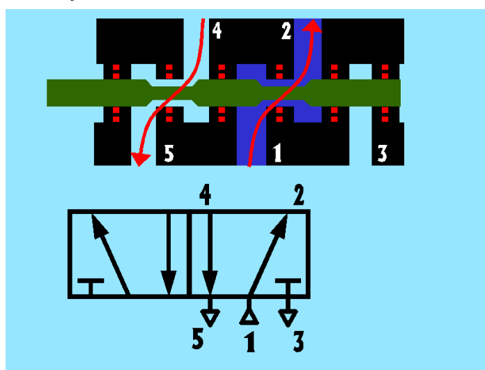
5/2-cestný ventil
