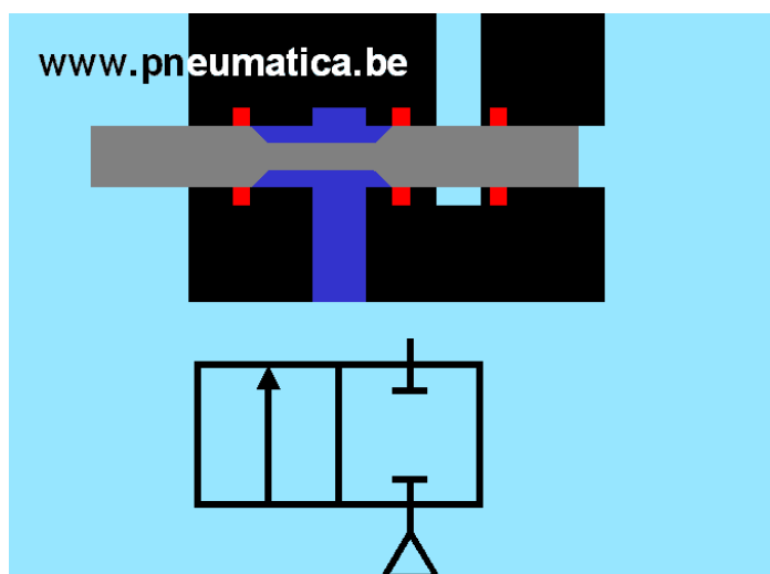
2/2-cestný ventil
