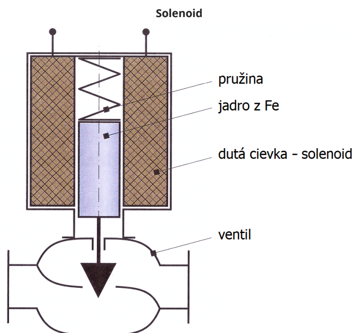
Solenoidový ventil
