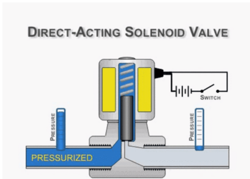
Sedlový ventil
