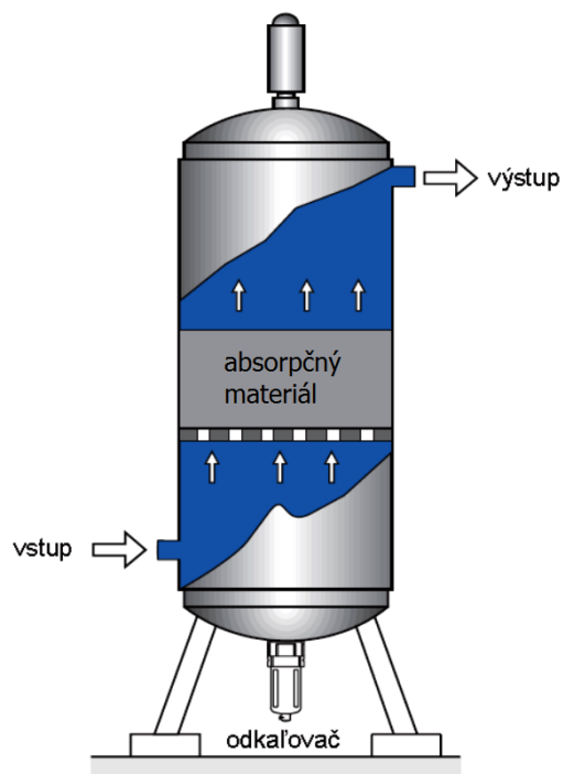
Absorpčná sušička podrobne
