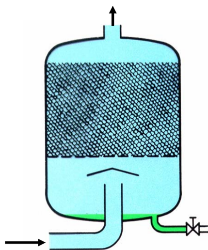
Princíp absorpčnej sušičky
