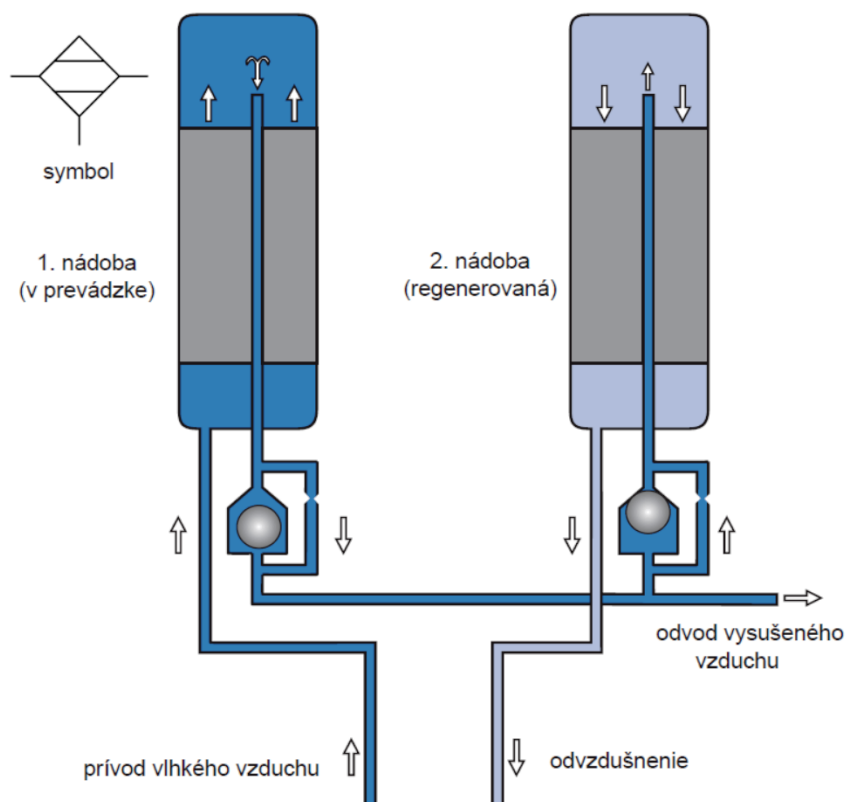
Adsorpčná sušička podrobne
