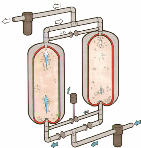
Princíp adsorpčnej sušičky
