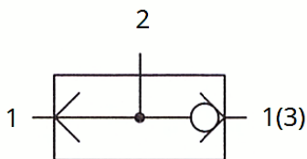
Značka trojcestného ventilu
