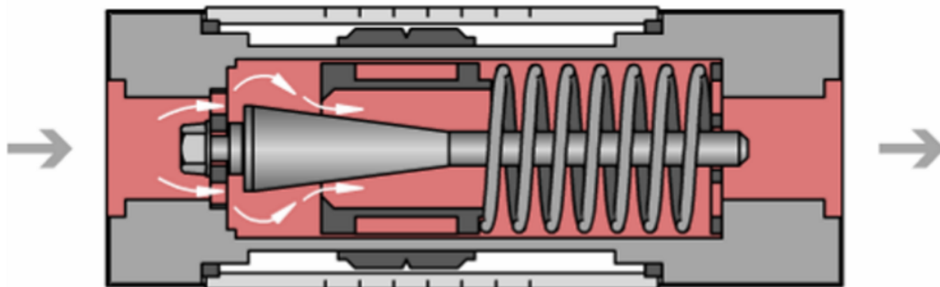
Prierez plavákového prietokomeru
