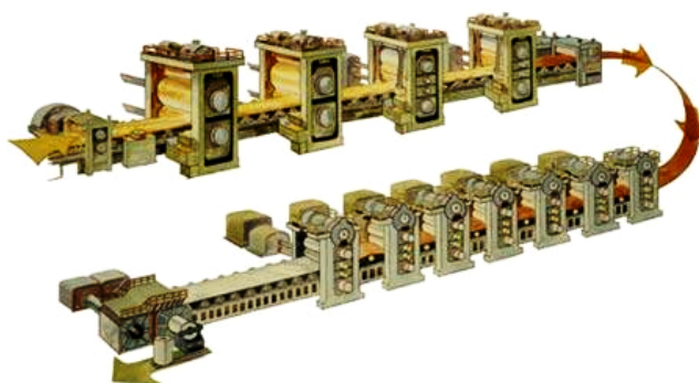
Valcovacia trať
