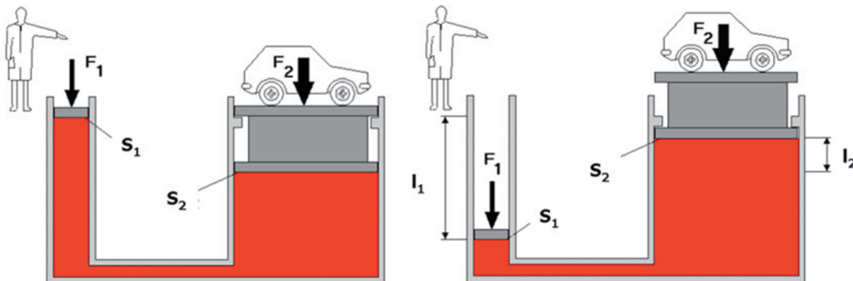
Dráhový prevod hydraulického mechanizmu
