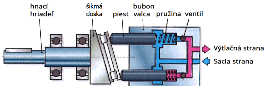
Zloženie - Čerpadlo so šikmou (výkyvnou) doskou
