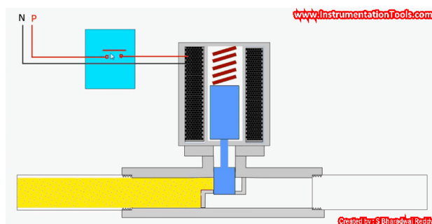
Riadenie sedlovým e-ventilom
