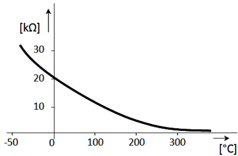
Charakteristika termistora
