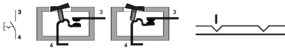
Svorka s aretáciou polohy (značka a princíp)
