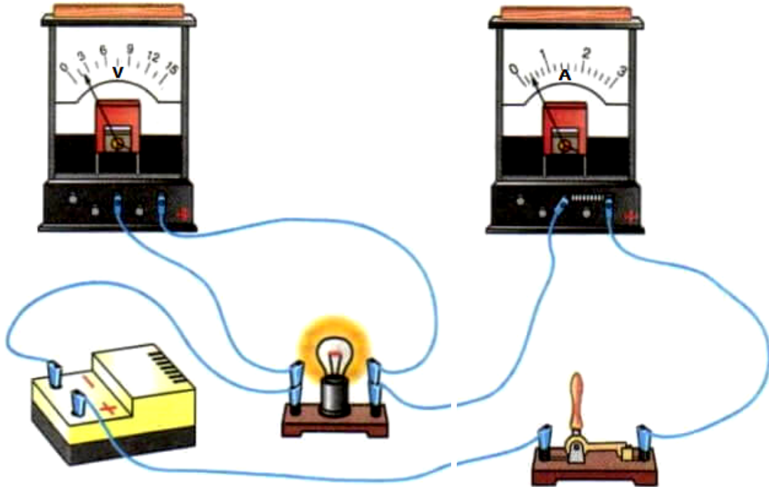
Meranie napätia a prúdu v elektrickom obvode
