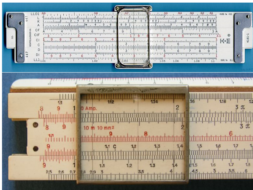
Logaritmičné pravítko
