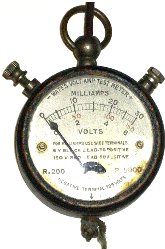
Multimeter z roku 1920
