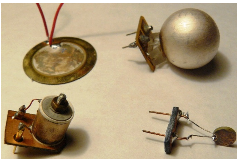
Rôzne tvary piezoelektrických snímačov
