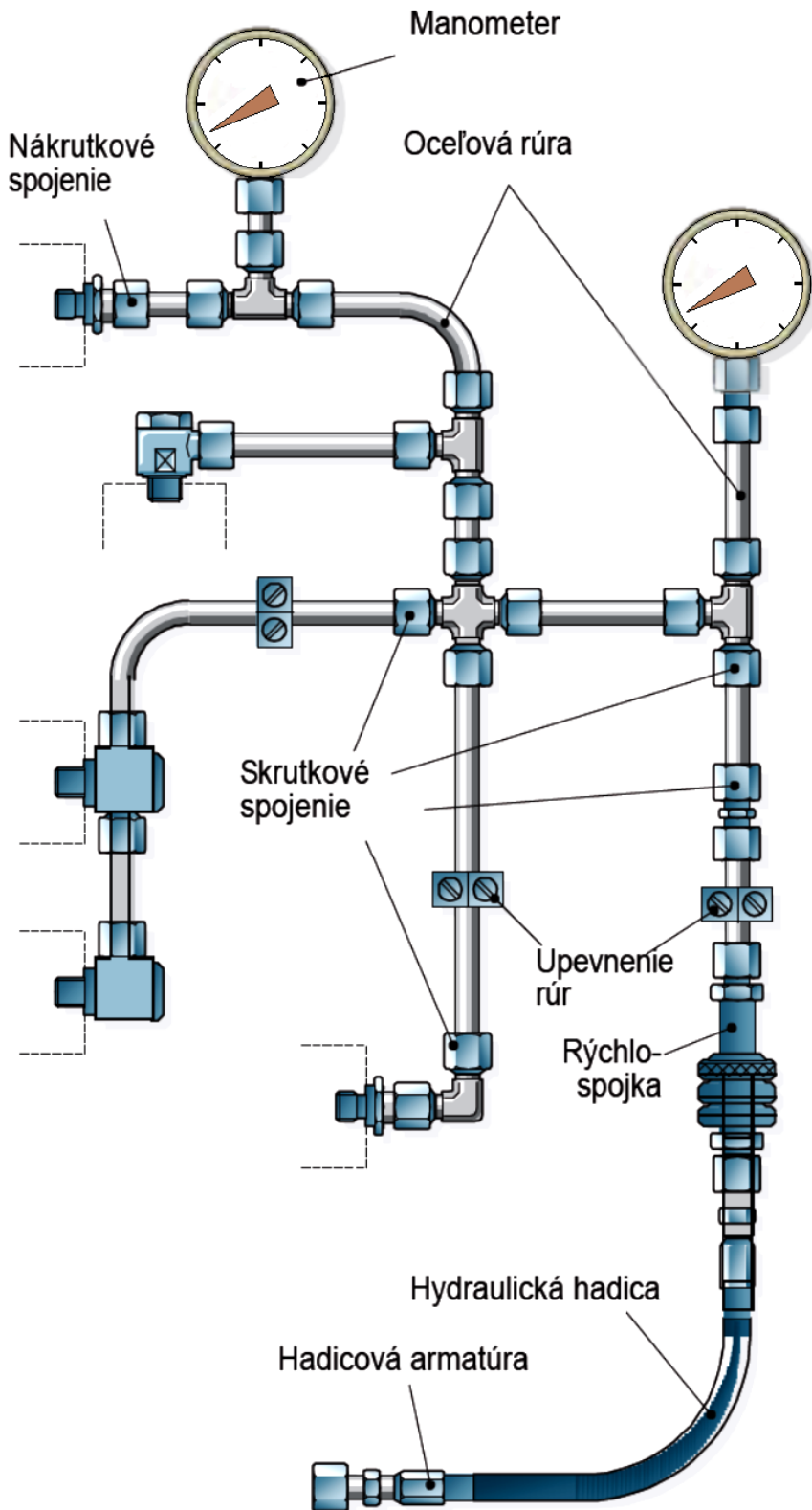
Potrubia a spojenie rúrok na závit
