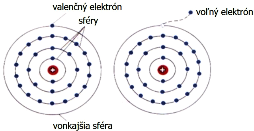
Model rozloženie elektrónov v elektrónovom obale medi
