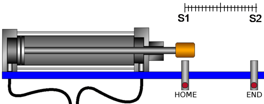
Dvojčinný valec a snímače koncovej polohy
