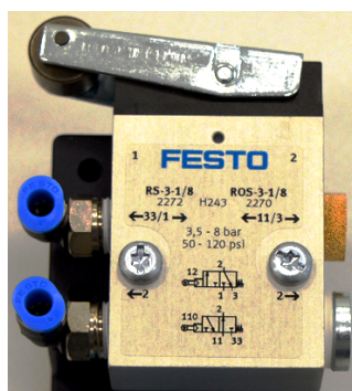
Mechanický koncový spínač
