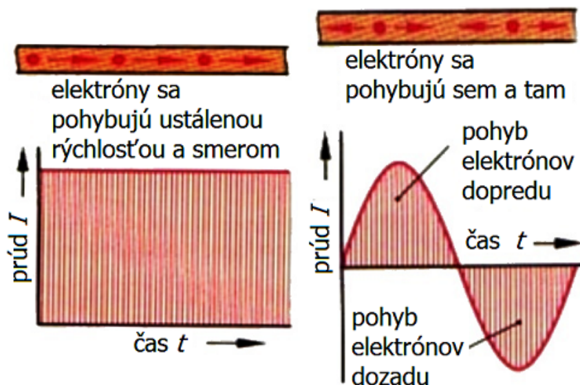
Grafické znázornenie jednosmerného a striedavého prúdu
