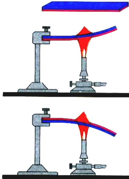
Bimetalický pásik: modrá - oceľ, purpurová - mosadz
