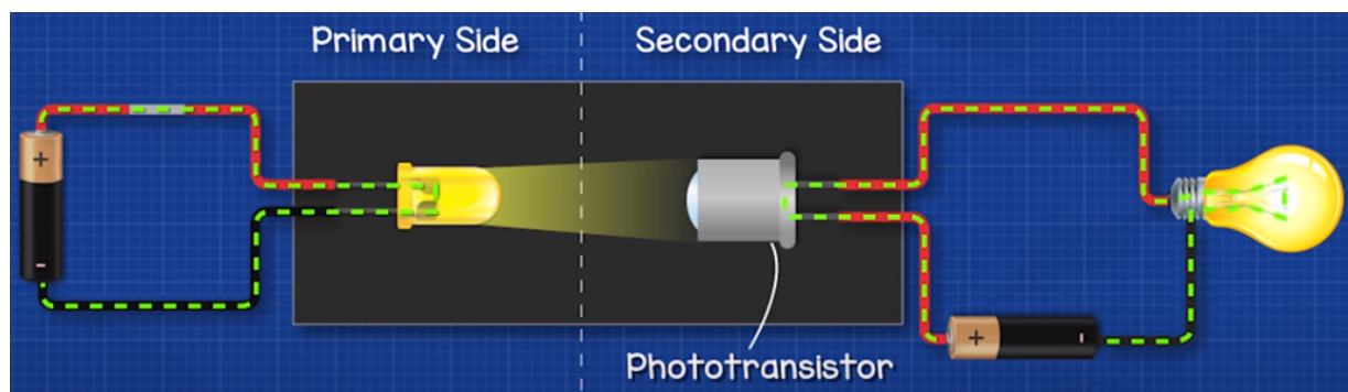
Princíp činnosti optrónu
