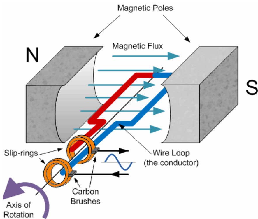
Vznik striedavého elektrického napätia a prúdu
