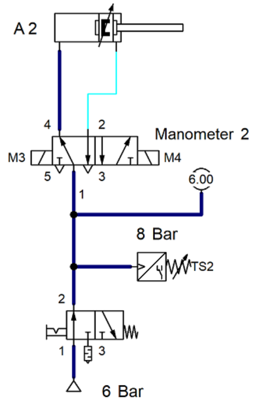
Zapojenie tlakového spínača nastaveného na tlak 8 barov. Spínač TS2 sa neaktivuje
